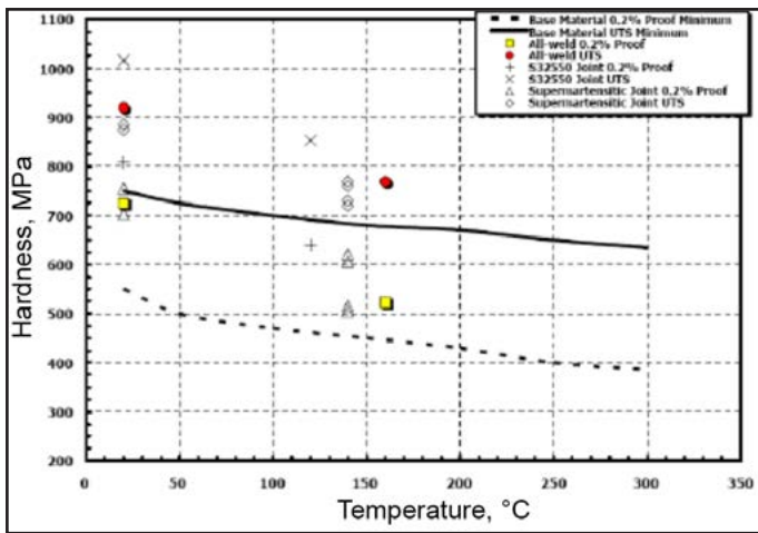
Fig 4. 150°C Tensile ER 25 9 4 CuWNL weld metal
